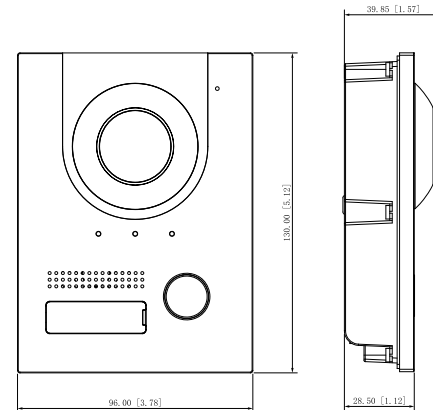
DHI-VTO2202F-P
